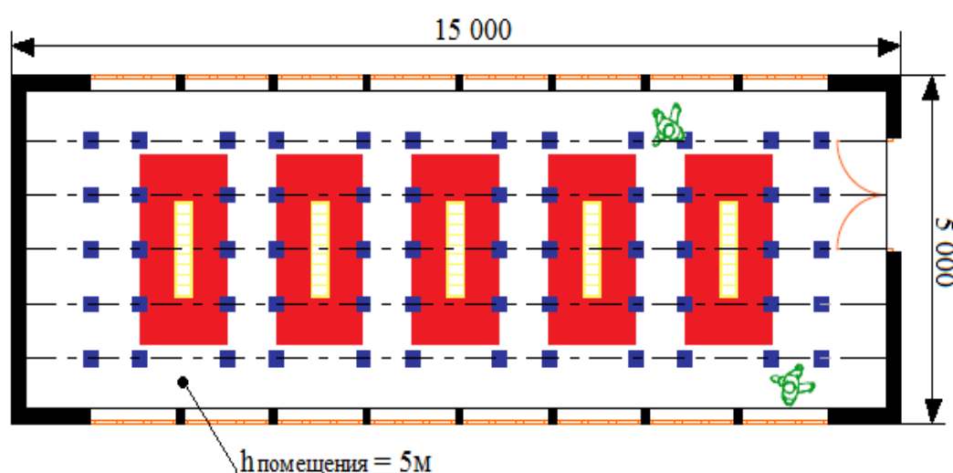
Рис. 4. План размещения объемных звукопоглотителей
