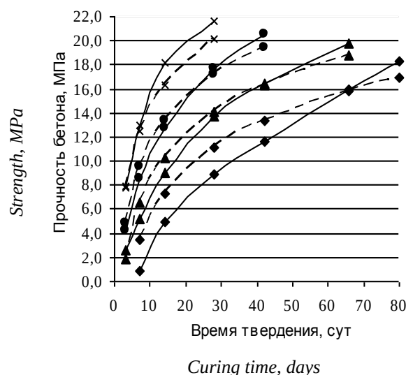
Рис. 5. Кинетика твердения бетона при пониженных температурах
