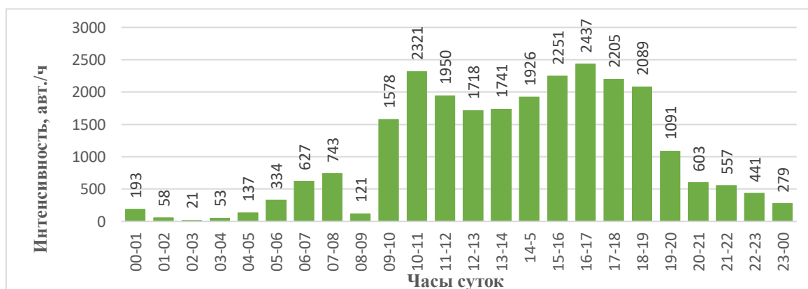
Рис. 2. Интенсивность движения 21.09.19
